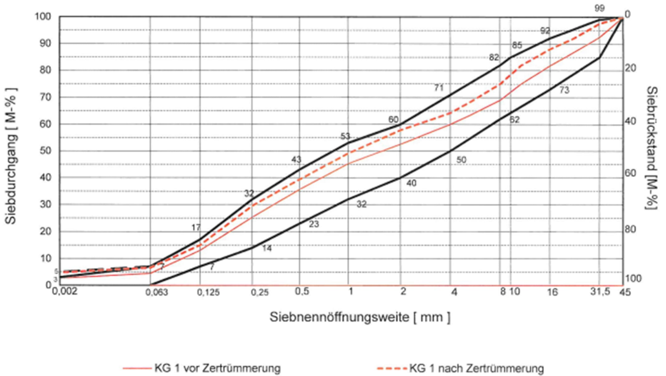
Sieblinienbereich für KG 1 (0/32) nach DBS 918 062
